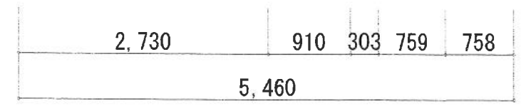
1階 平面図 S:1/60
